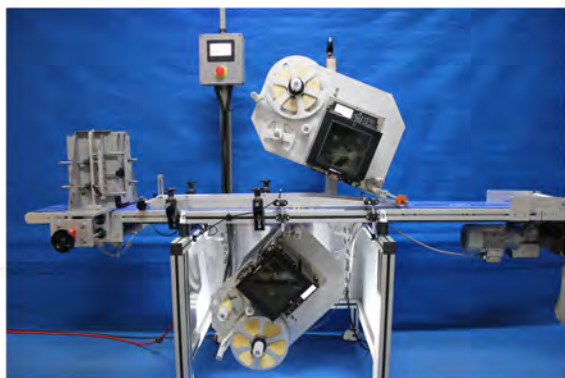
Étiqueteuse Dessus-Dessous avec dépileur de sachets
